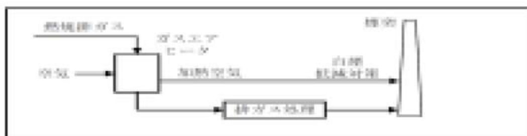
図2 熱回収設備(2)
